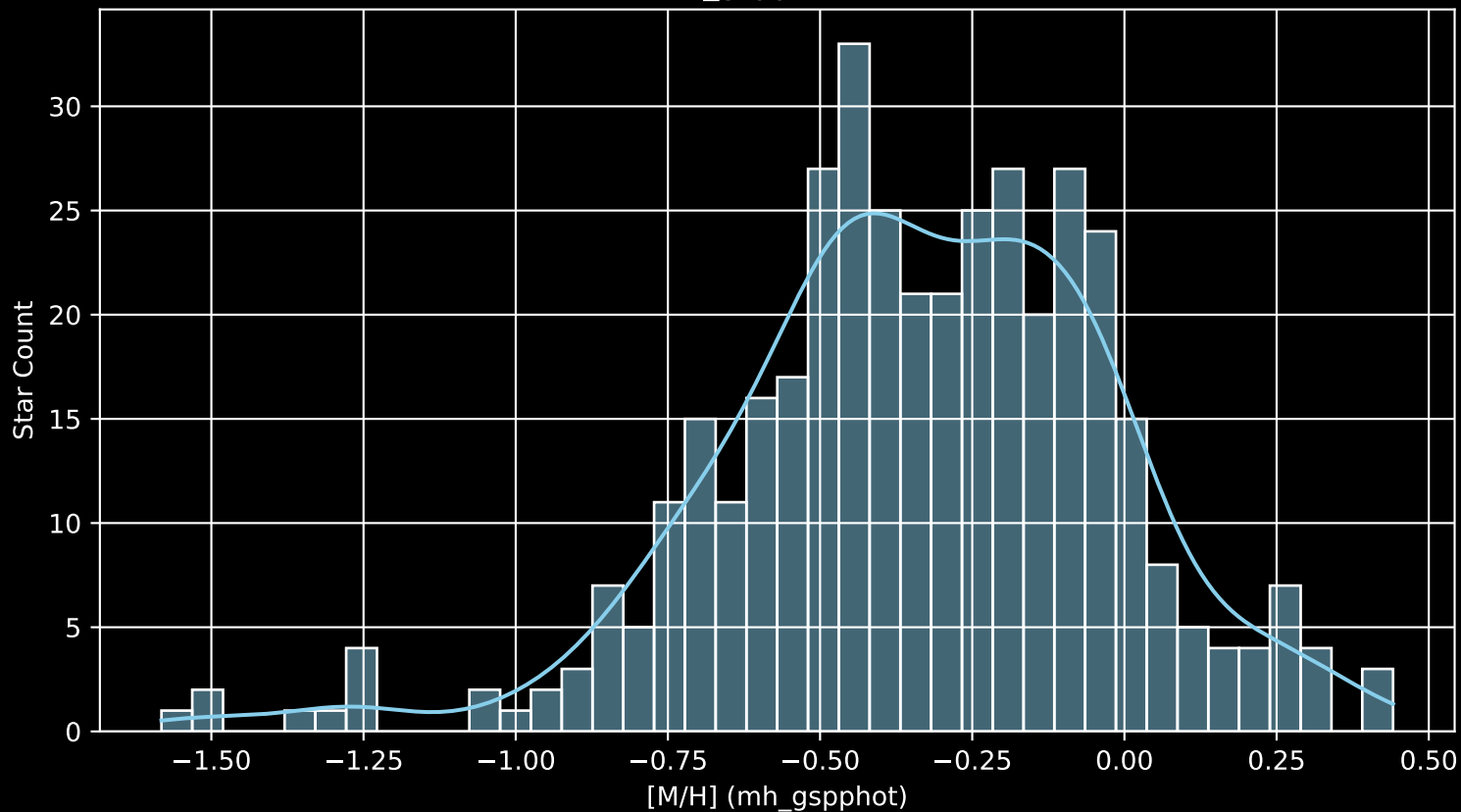
GALAH DR4 Field: [6685] [M/H] (mh_gspphot) (n= 399)
