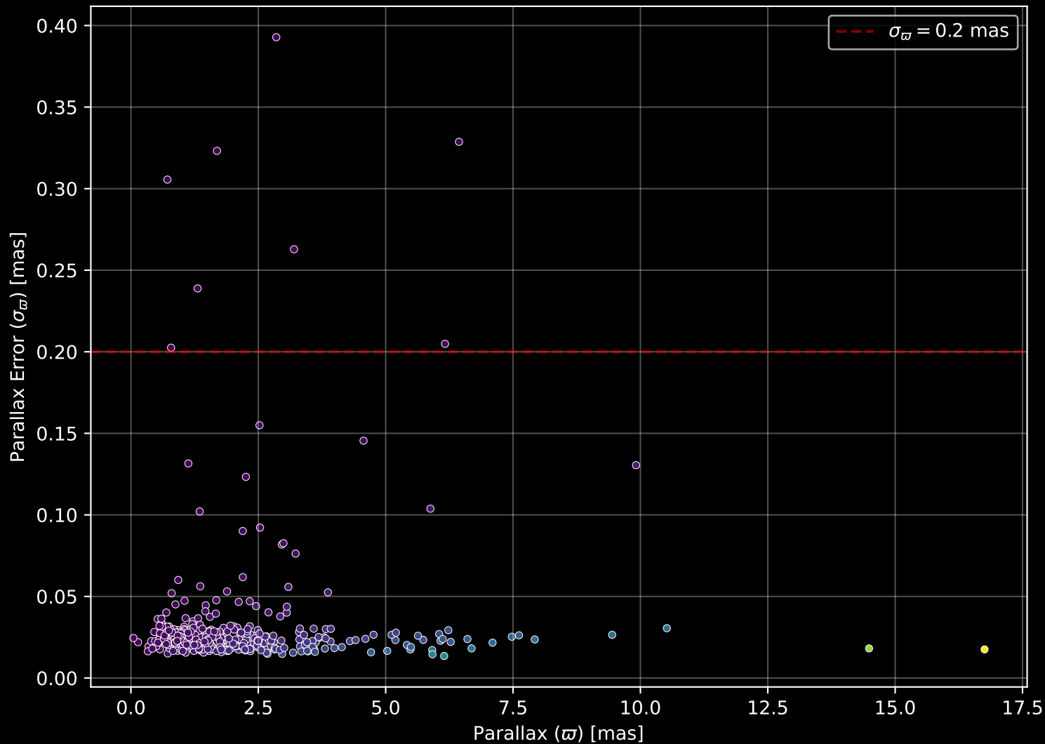
GALAH DR4 Field: [6685] Parallax Quality (n= 402)
