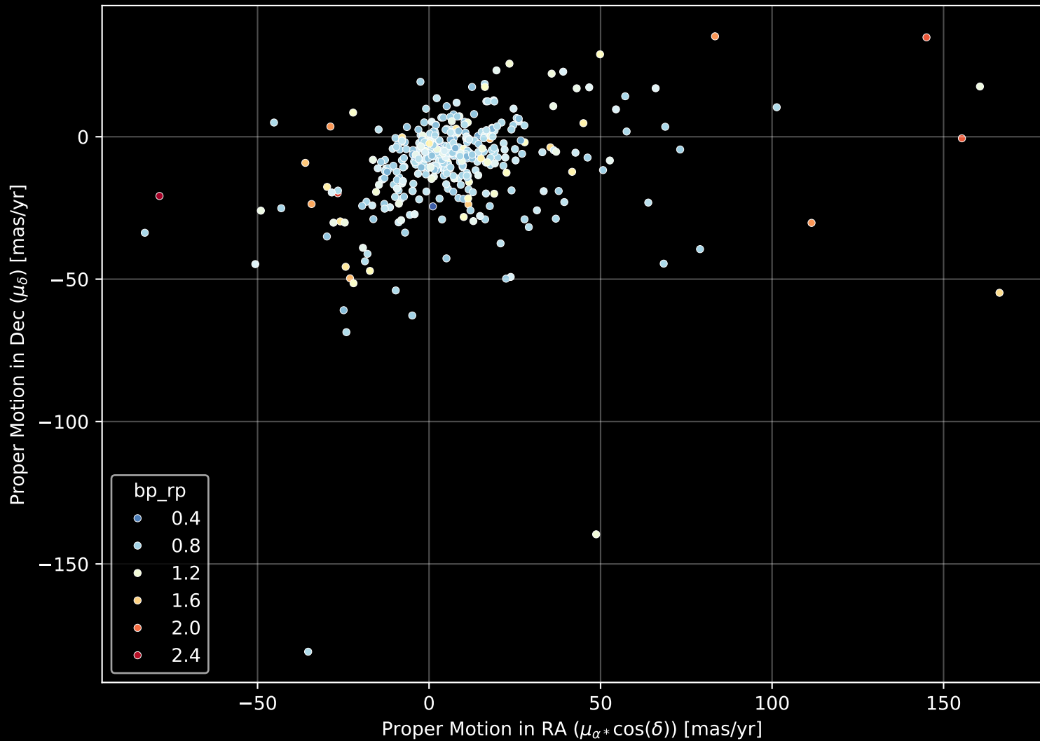
GALAH DR4 Field: [6685] Proper Motion Diagram (n= 402)
