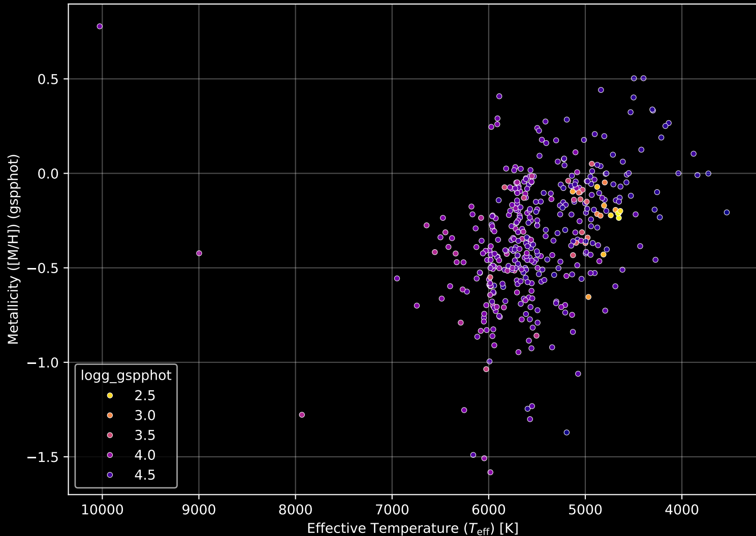
GALAH DR4 Field: [6685] Stellar Population Parameters (n= 402)
